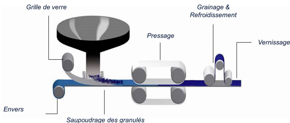
Figure 5 : Illustration d'un process de Pressage
