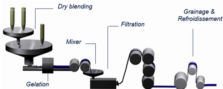
Figure 4 : Illustration d'un process de Calandrage
